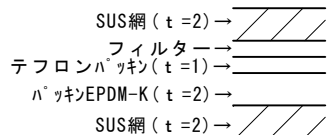
D 拡大図 (吐出部)
