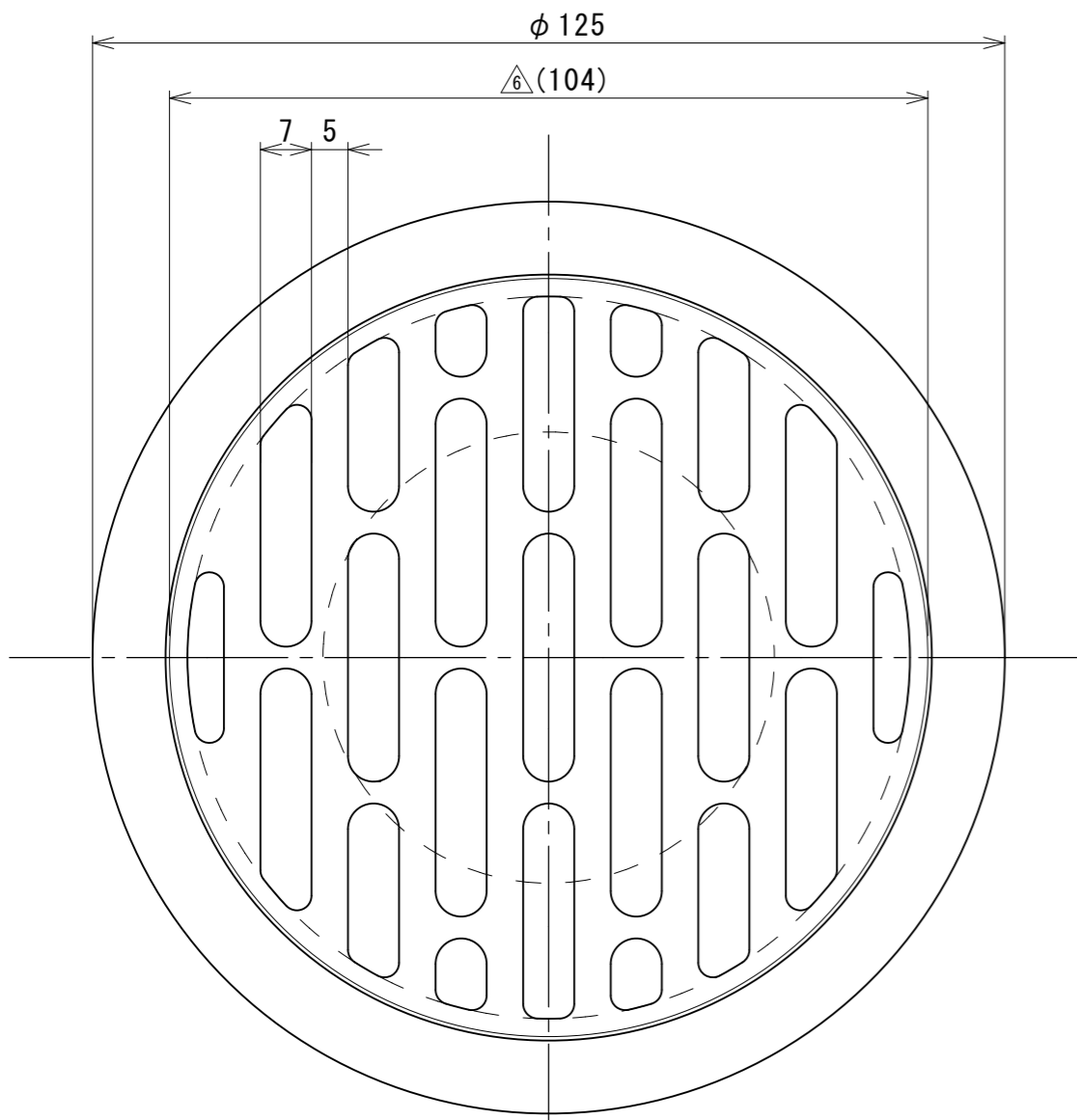
平面図
