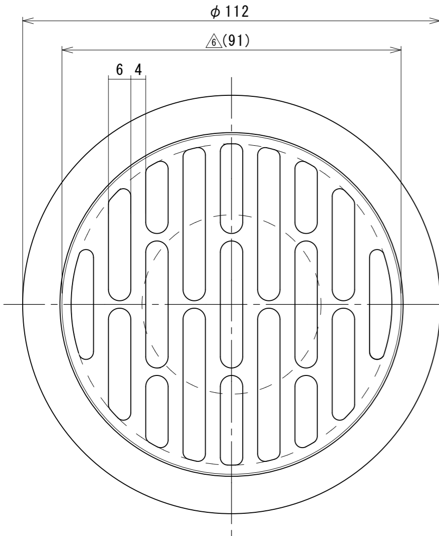
平面図
