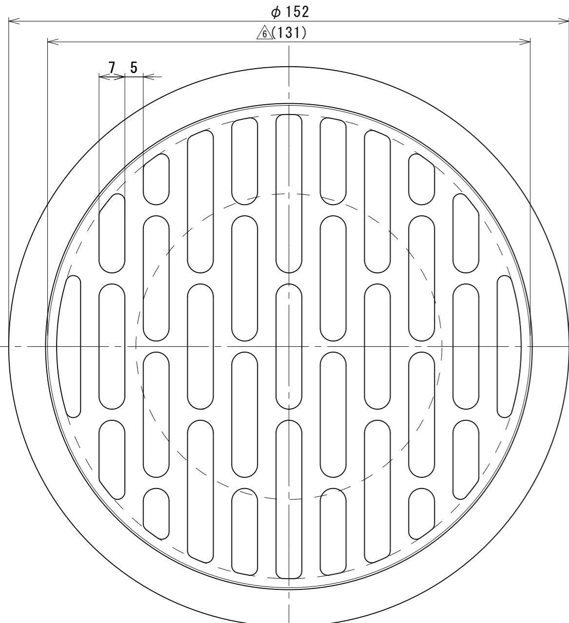
平面図
