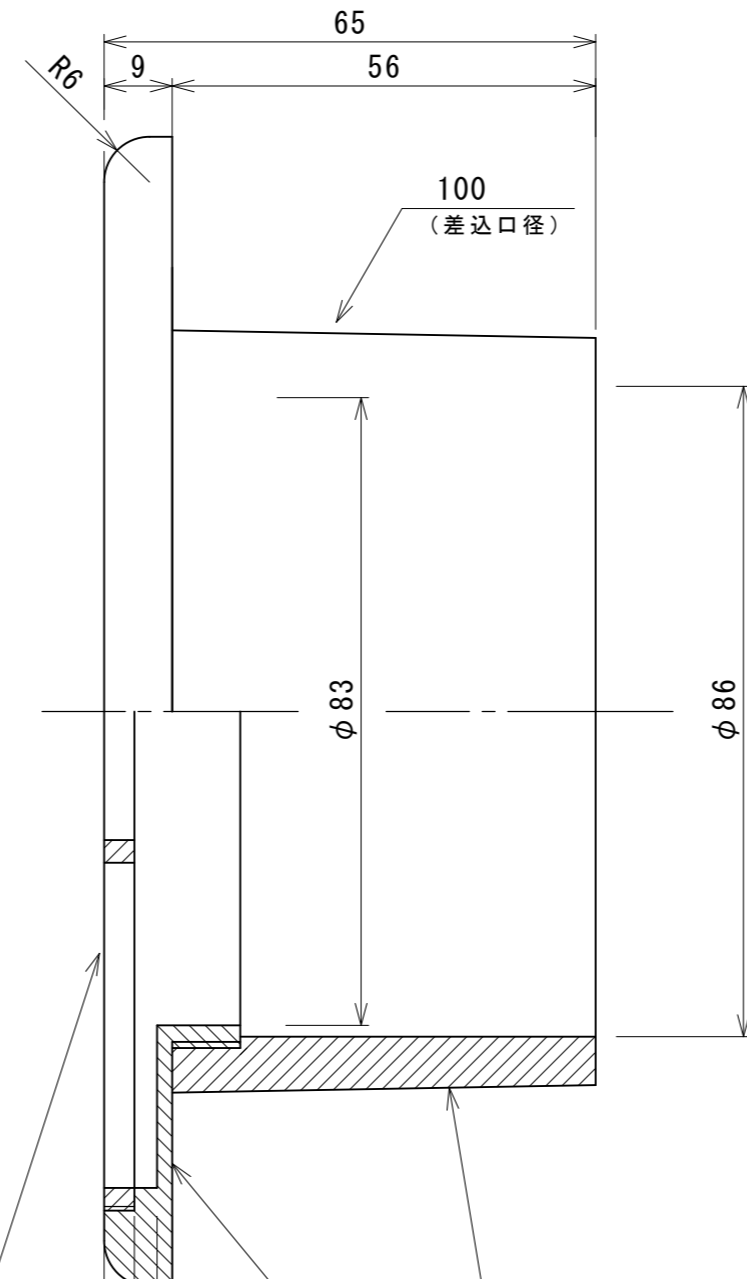
断側面図
