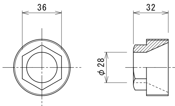
② オリフィス部品図
