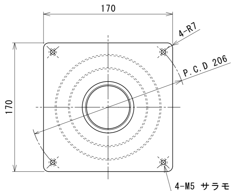
B 矢視図
