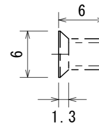
SNFS-SD M4 x 6L 固定ボルト詳細図 S=NON
