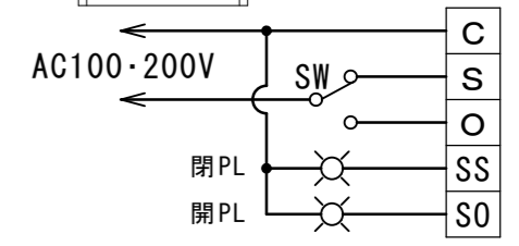
結線図
